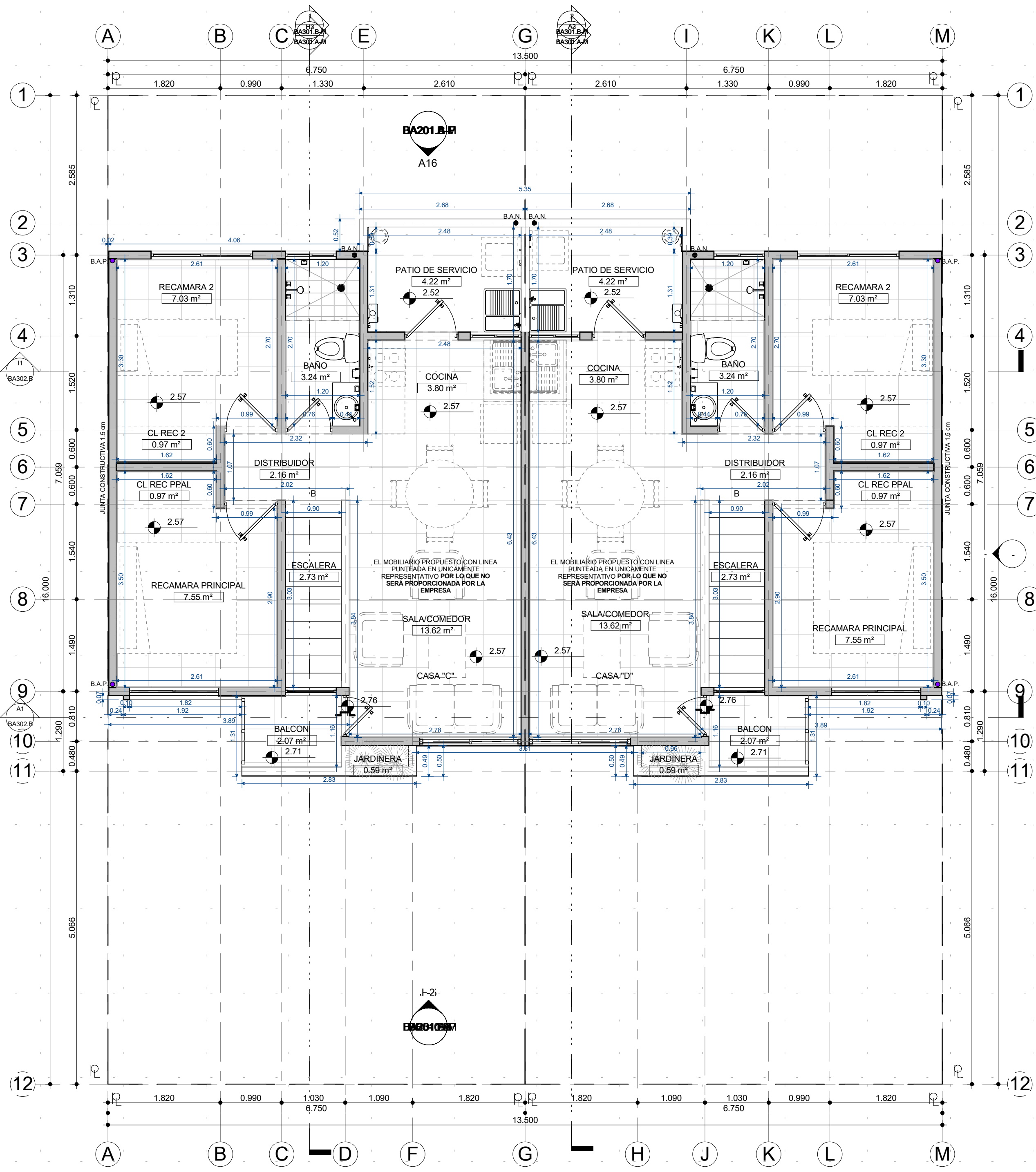
A1 ARQ PLANTA ALTA OPCION "B" 1:50
